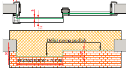
Dveře posuvné s bočním světlíkem – obložková konstrukce
